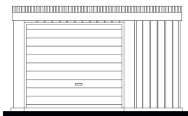
ELEWACJA FRONTOWA
