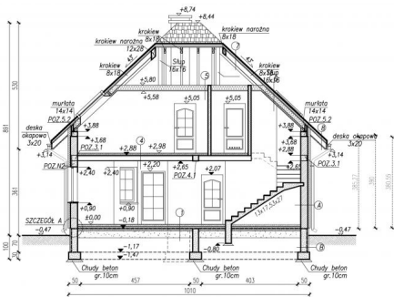
PRZEKRÓJ B-B
