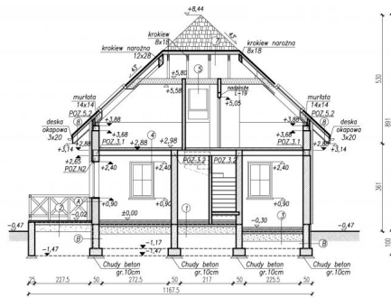
PRZEKRÓJ B-B
