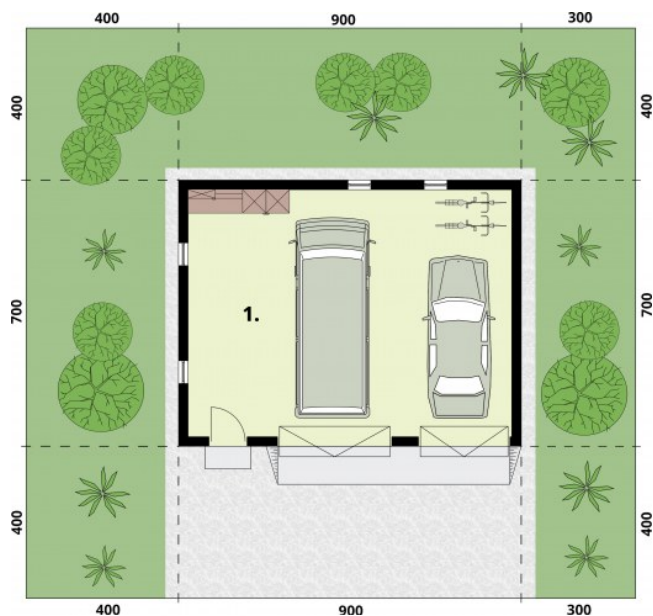
Rzut przyziemia
