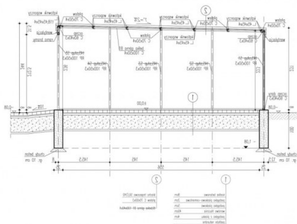
Przekrój
