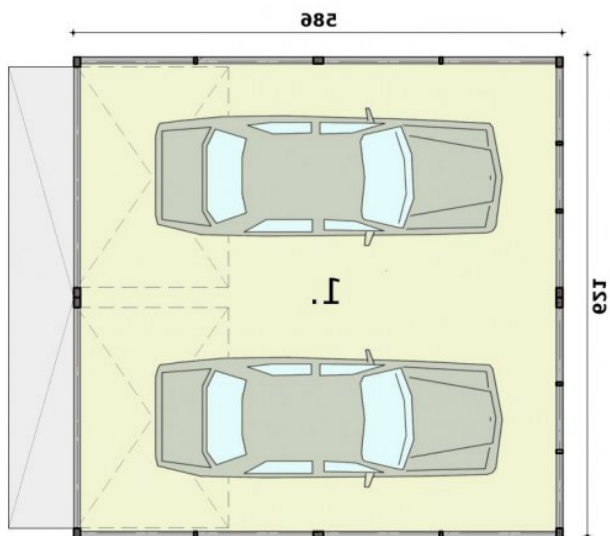
Rzut przyziemia
