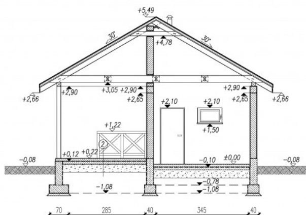
PRZEKRÓJ B-B
