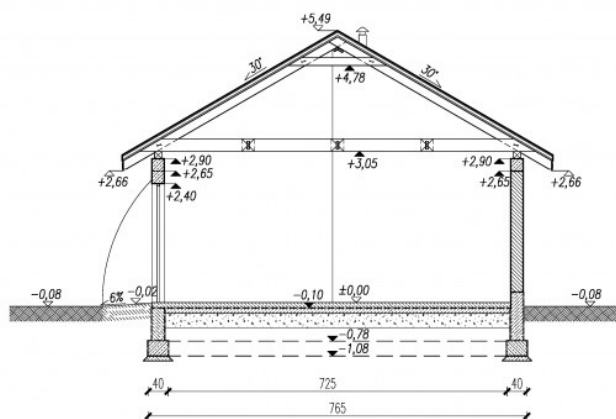
PRZEKRÓJ B-B
